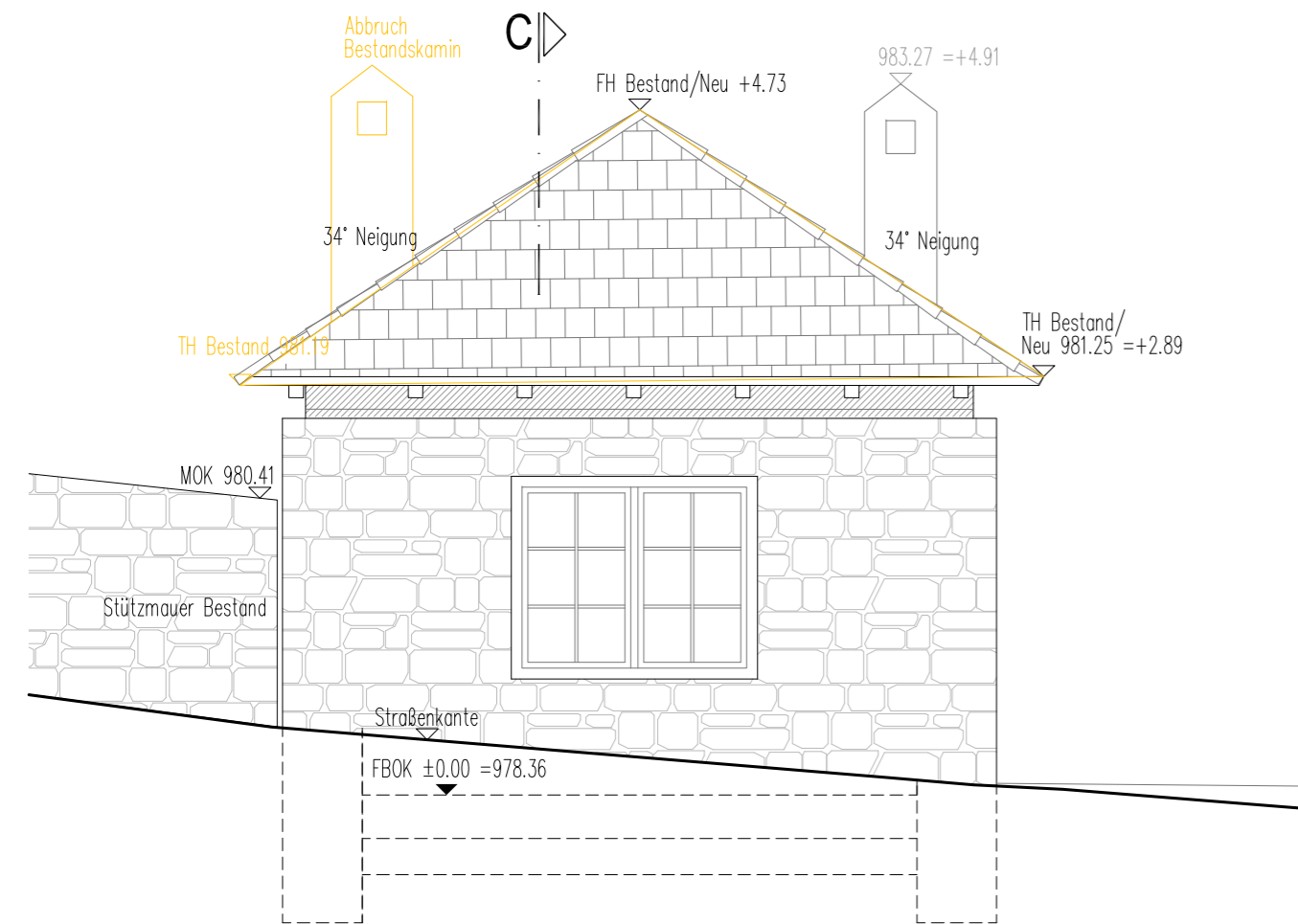
Ansicht Südwest
