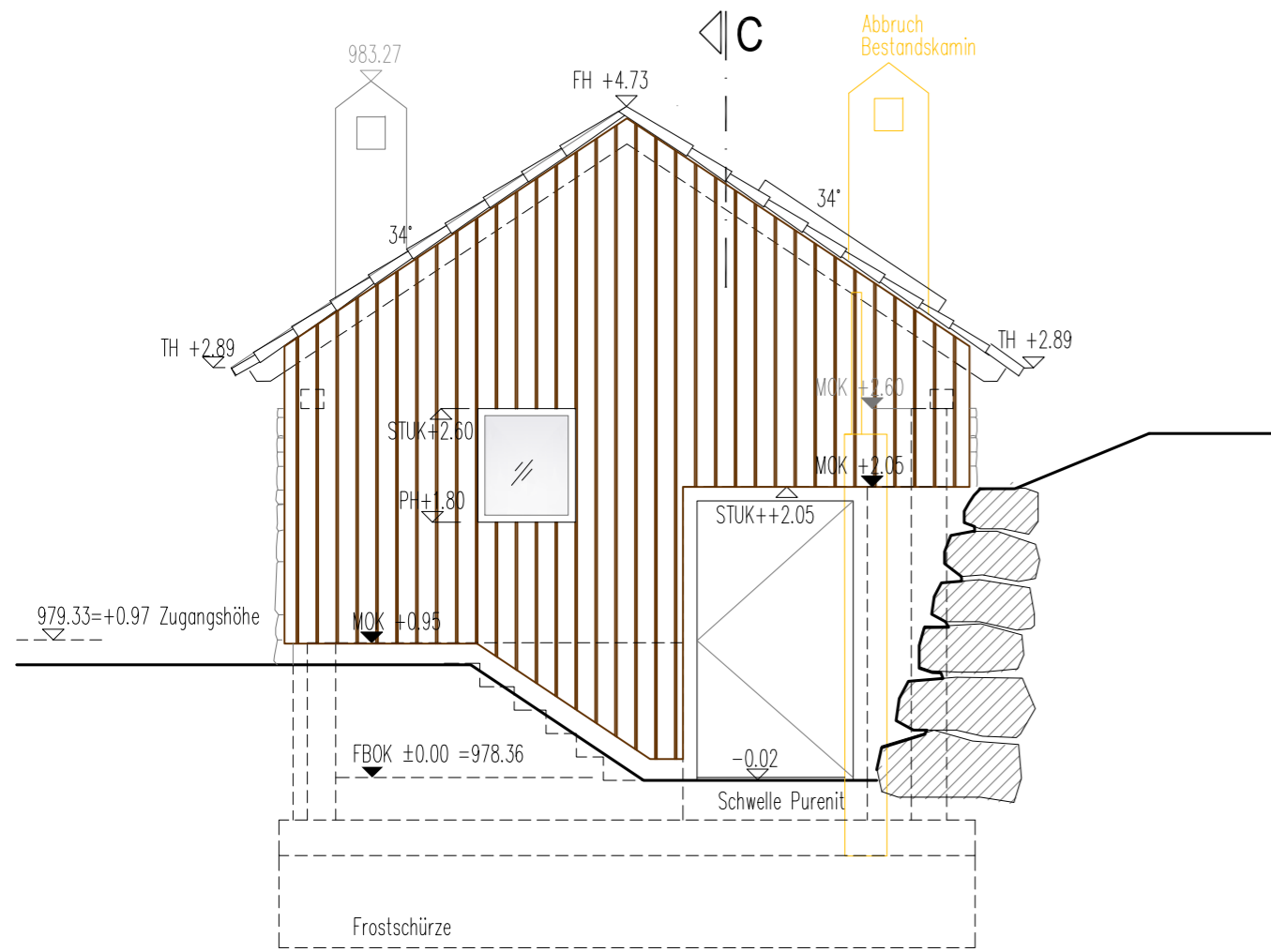
Ansicht Nordost
