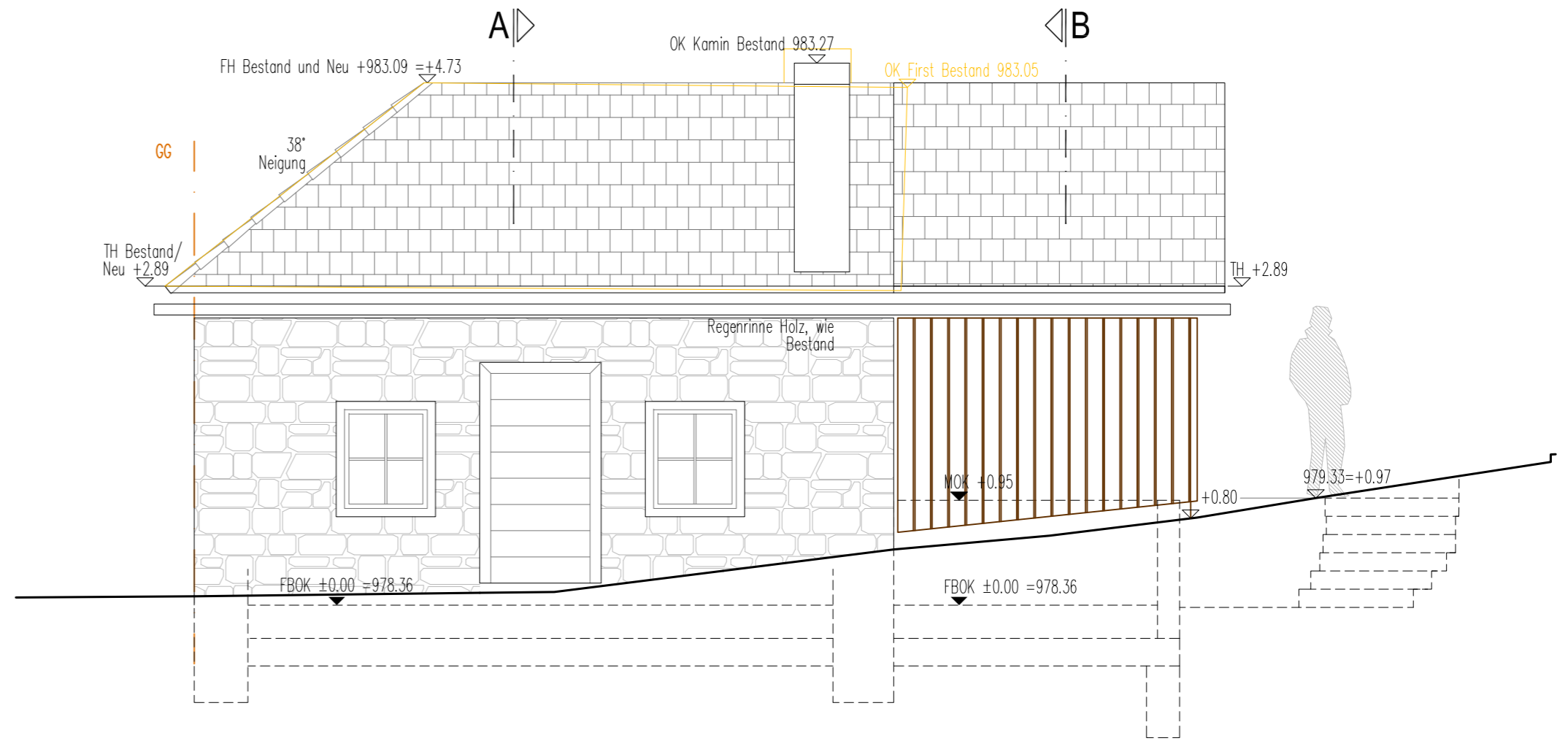
Ansicht Südost
